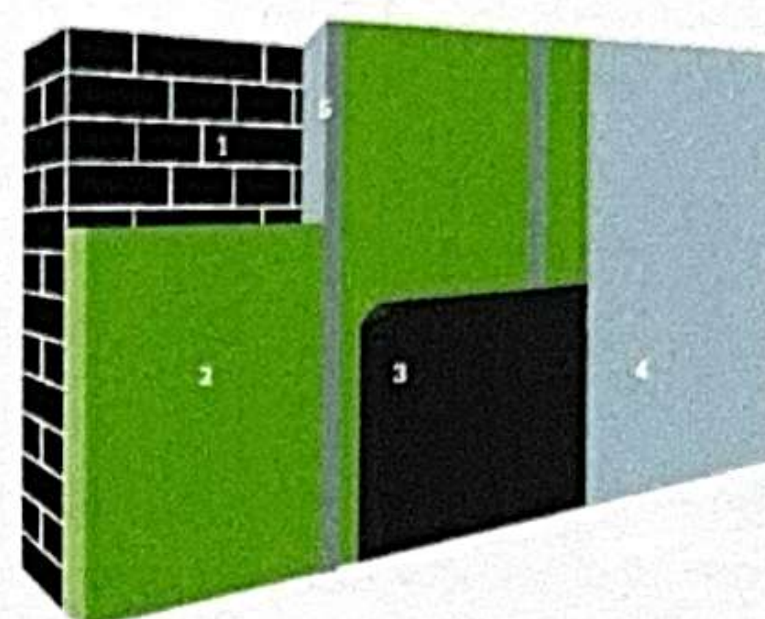
1. Buitengevel | 2. Isolatie | 3. Dampschermb | 4. Binnenafwerking | 5. Stijl- en regelwerk (optioneel)
