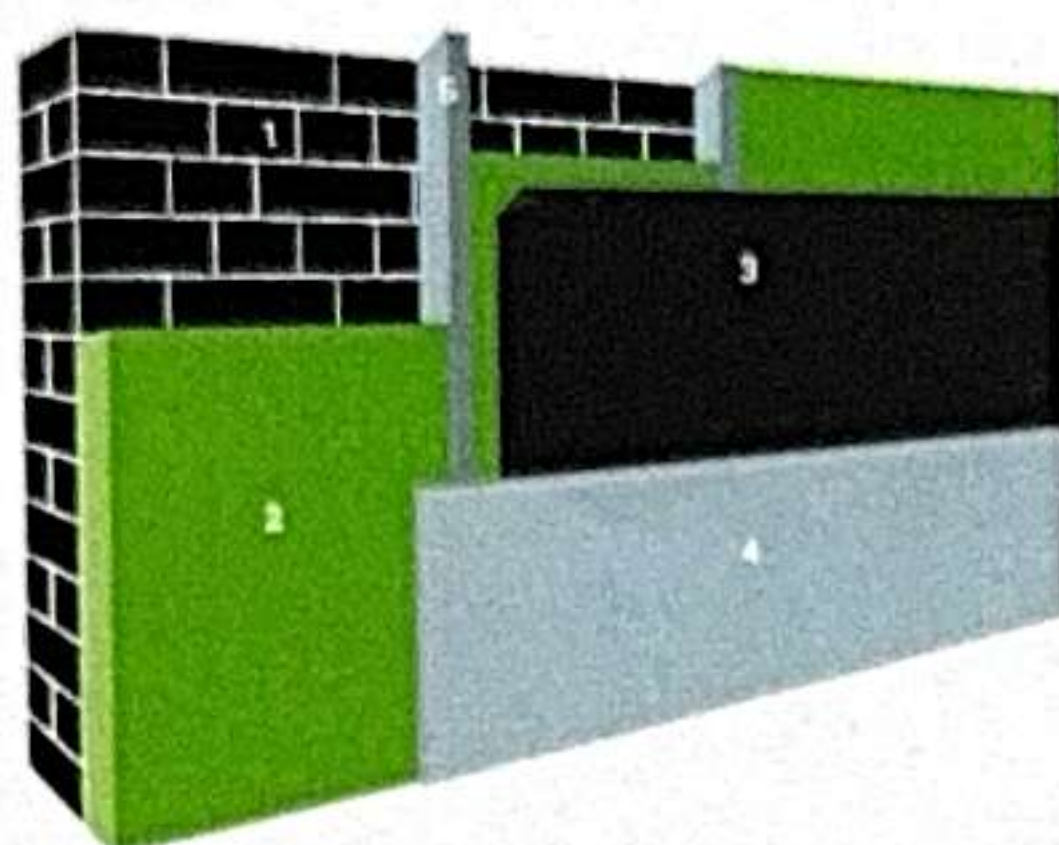
1. Buitenmuur | 2. Isolatie | 3. Vochtschermb | 4. Afwerkingslaag | 5. Stijl- en regelwerk (optioneel)
